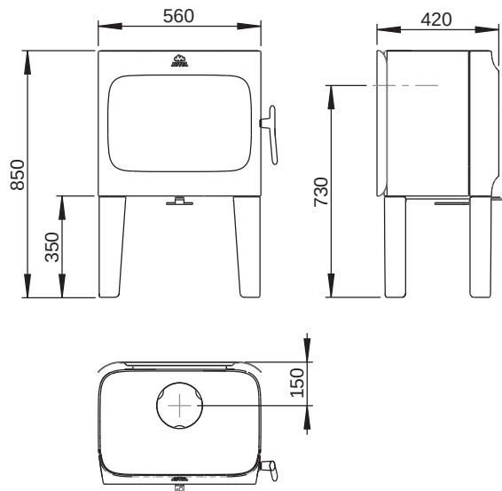
Jøtul F 305 LL (Lange ben)
