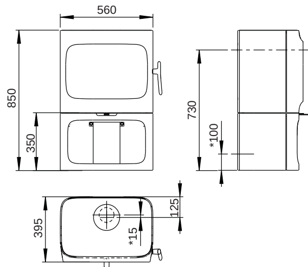
Jøtul F 305 R B (med sokkel)
