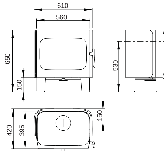
Jøtul F 305 C SL (korte ben)
