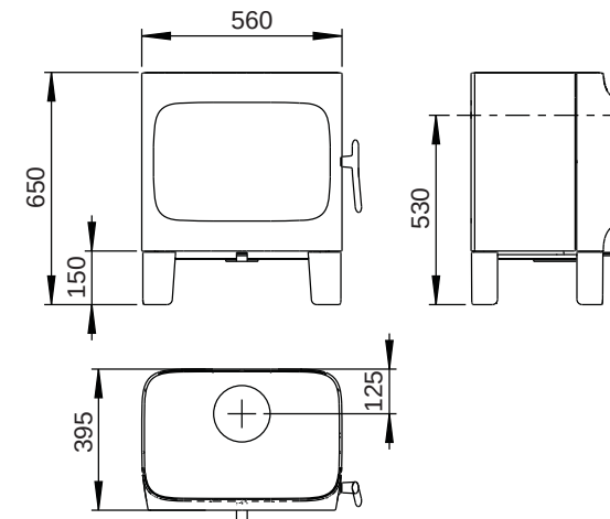
Jøtul F 305 R SL (korte ben)
