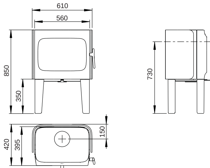
Jøtul F 305 C LL (lange ben)
