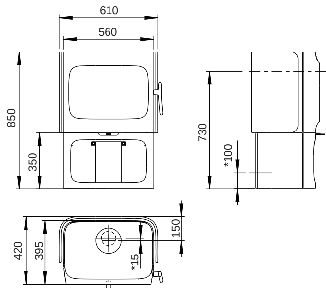
Jøtul F 305 C B (sokkel)
