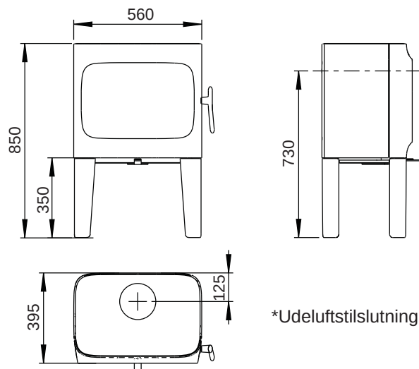
Jøtul F 305 R LL (lange ben)
