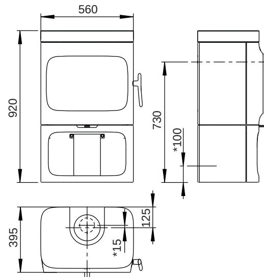
Jøtul F 305 R B (med sokkel og fedtstenstop)
