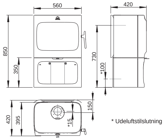
Jøtul F 305 B (sokkel)
