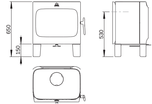
Jøtul F 305 SL (korte ben)
