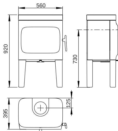
Jøtul F 305 R LL (lange ben og fedtstenstop)
